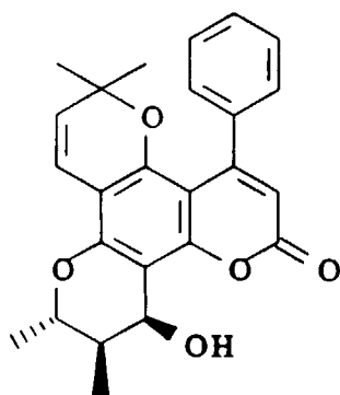
SOULATTROLIDE
