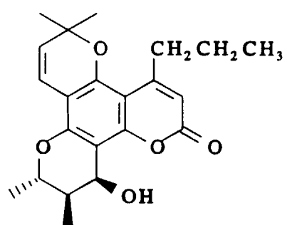
COSTATOLIDE
