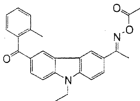
IRGACURE OXE 02
