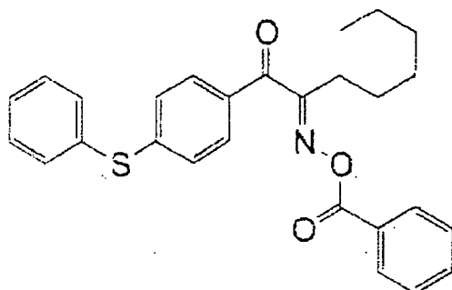
IRGACURE OXE 01
