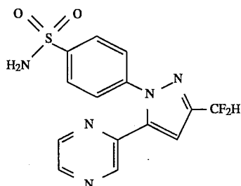
4-[5-(4-Pyrazinyl)-3-(difluoromethyl)-1H-pyrazol-1-yl]benzenesulfonamide
