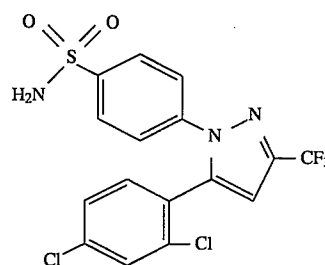
4-[5-(2,4-Dichlorophenyl)-3-(trifluoromethyl)-1H-pyrazol-1-yl]benzenesulfonamide
