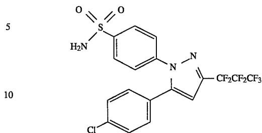
4-[5-(4-Chlorophenyl)-3-(heptafluoropropyl)-1H-pyrazol-1-yl]benzenesulfonamide
