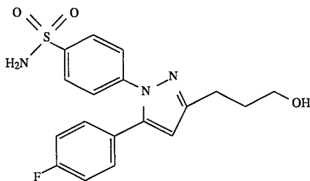
4-[5-(4-Fluorophenyl)-3-(3-hydroxypropyl)-1H-pyrazol-1-yl]benzenesulfonamide
