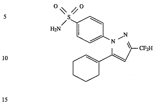
4-[5-(1-Cyclohexenyl)-3-(difluoromethyl)-1H-pyrazol-1-yl]benzenesulfonamide
