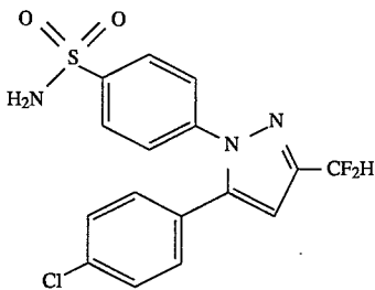
4-[5-(4-Chlorophenyl)-3-(difluoromethyl)-1H-pyrazol-1-yl]benzenesulfonamide
