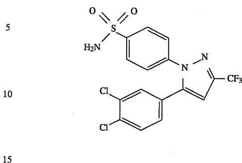
4-[5-(3,4-Dichlorophenyl)-3-(trifluoromethyl)-1H-pyrazol-1-yl]benzenesulfonamide
