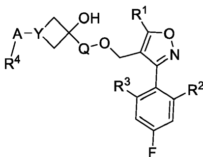
(Ia)
