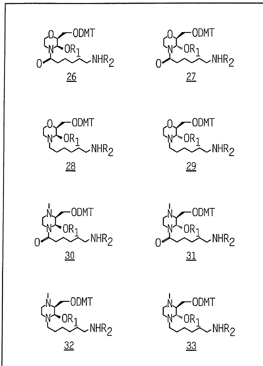
FIG. 3C
