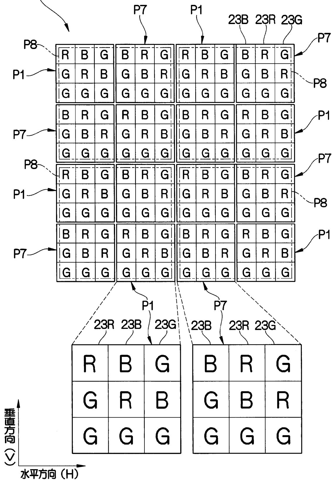
50 (カラーフィルタ配列)
