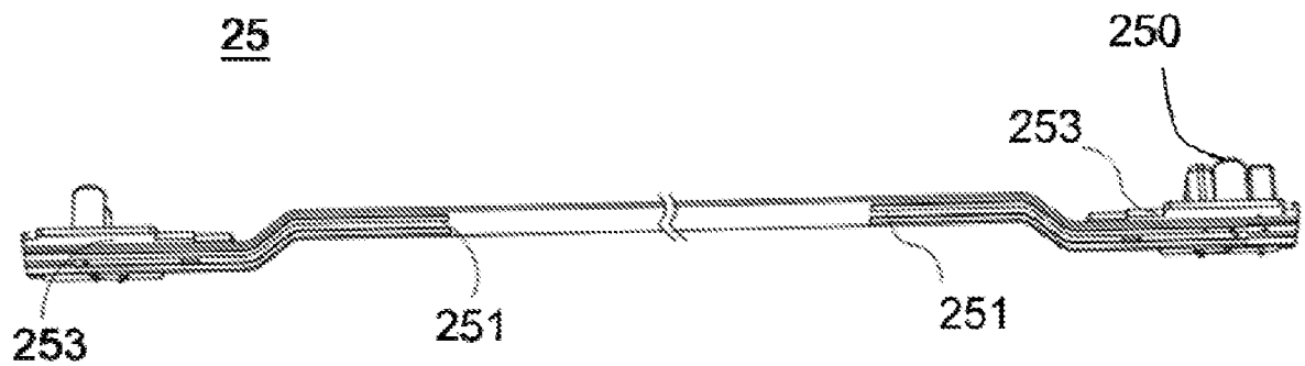
Fig. 36
