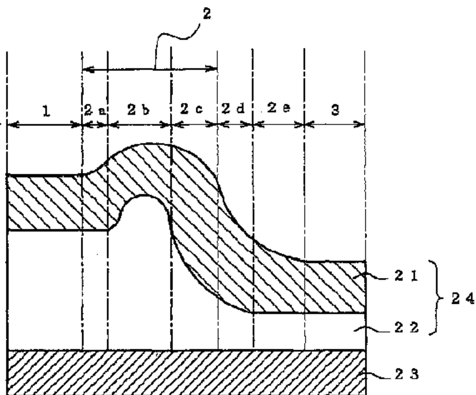
section A-A'
