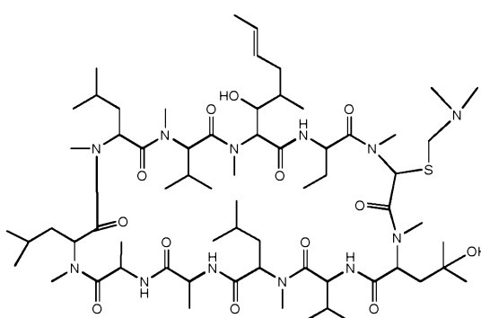
SCY-635, 4
