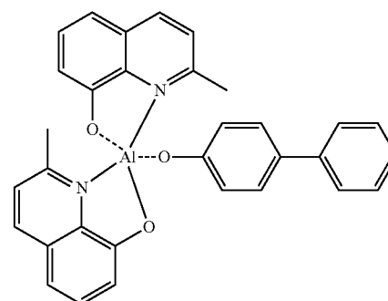
BAlq
