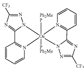
Os(fptz) 2 (PPh 2 Me) 2
