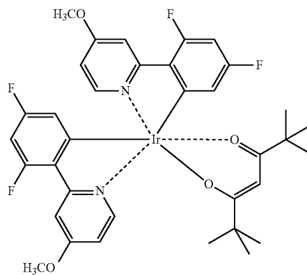
(F_2ppy)_2Ir(tmd)
