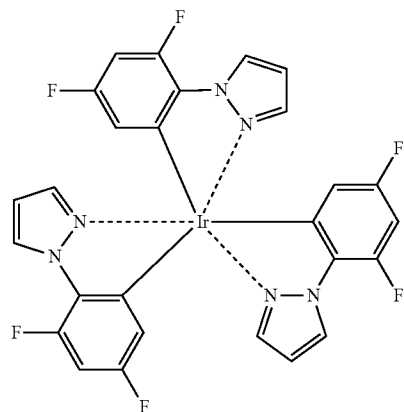
Ir(dfppz)_3
