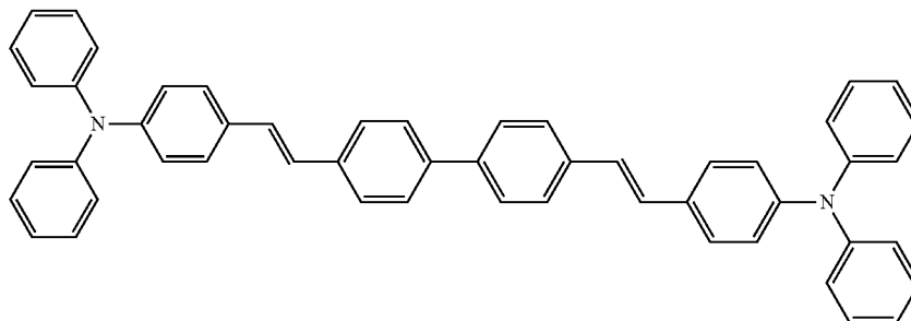
DPAVBi
