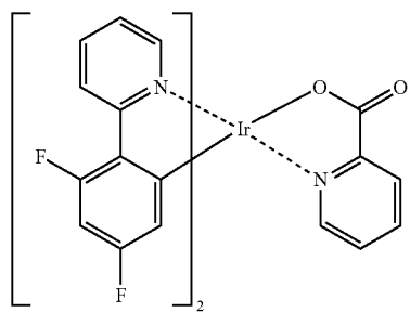
F_2Irpic
