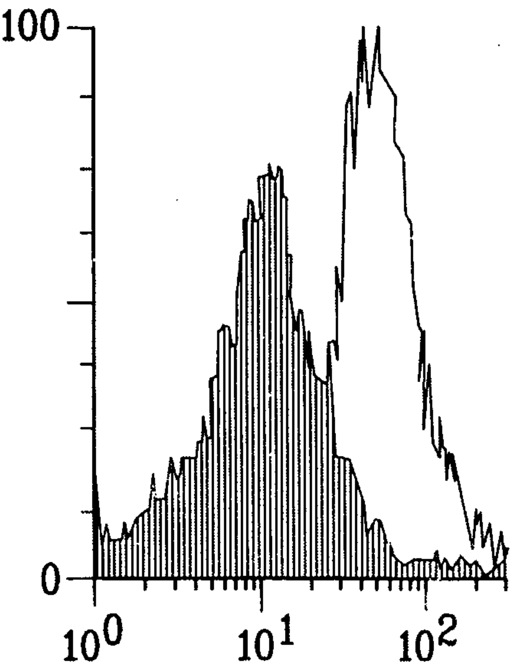
FIG. 7C 206 (17 kDa) FACS
