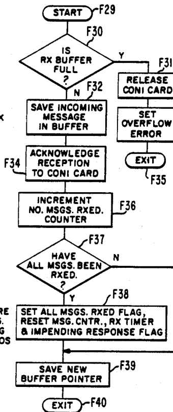
FIG. 25 GET RX MESSAGE
