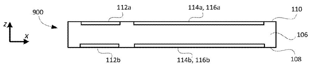
FIG. 9A (top view)
