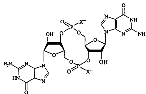
c-GpXGpX X = S, Se stereochemically pure (VI)
