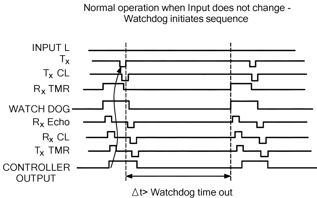
FIG. 5C
