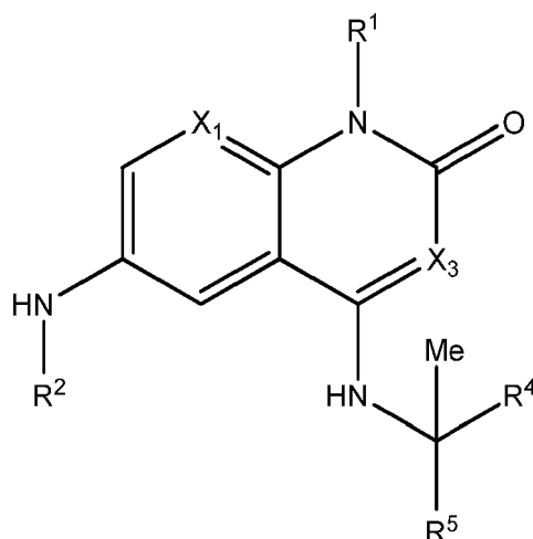
Formule Ib 2
