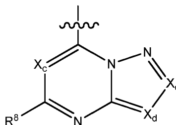
Formule B
