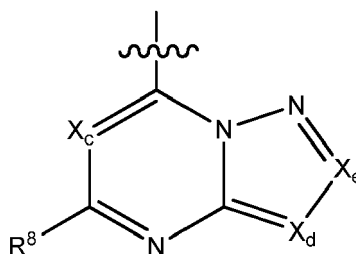
Formule B
