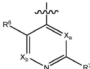
Formule A
