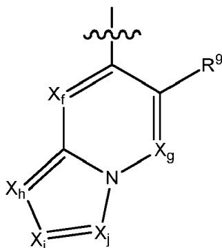
Formule C
