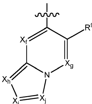
Formule C
