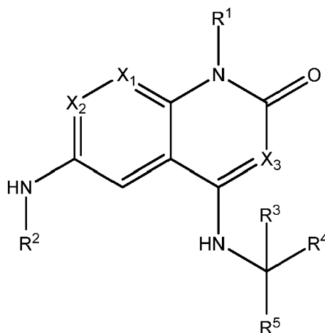
Formule (I)
