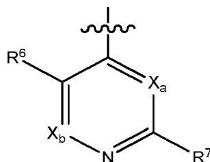
Formule A
