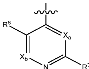
Formule A
