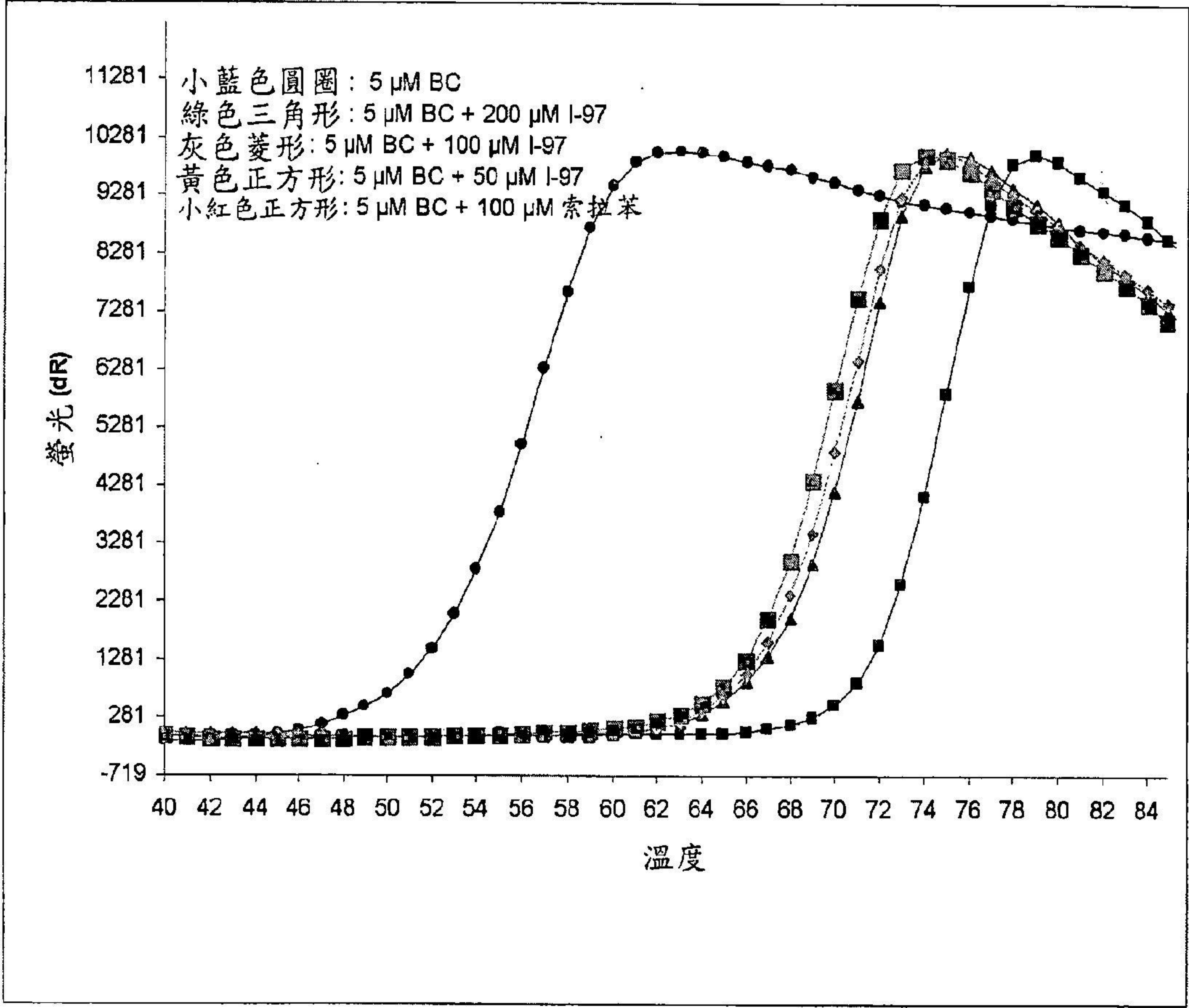
針對ACC2之生物素羧化酶結構域之化合物I-97之熱移變分析之結果。
