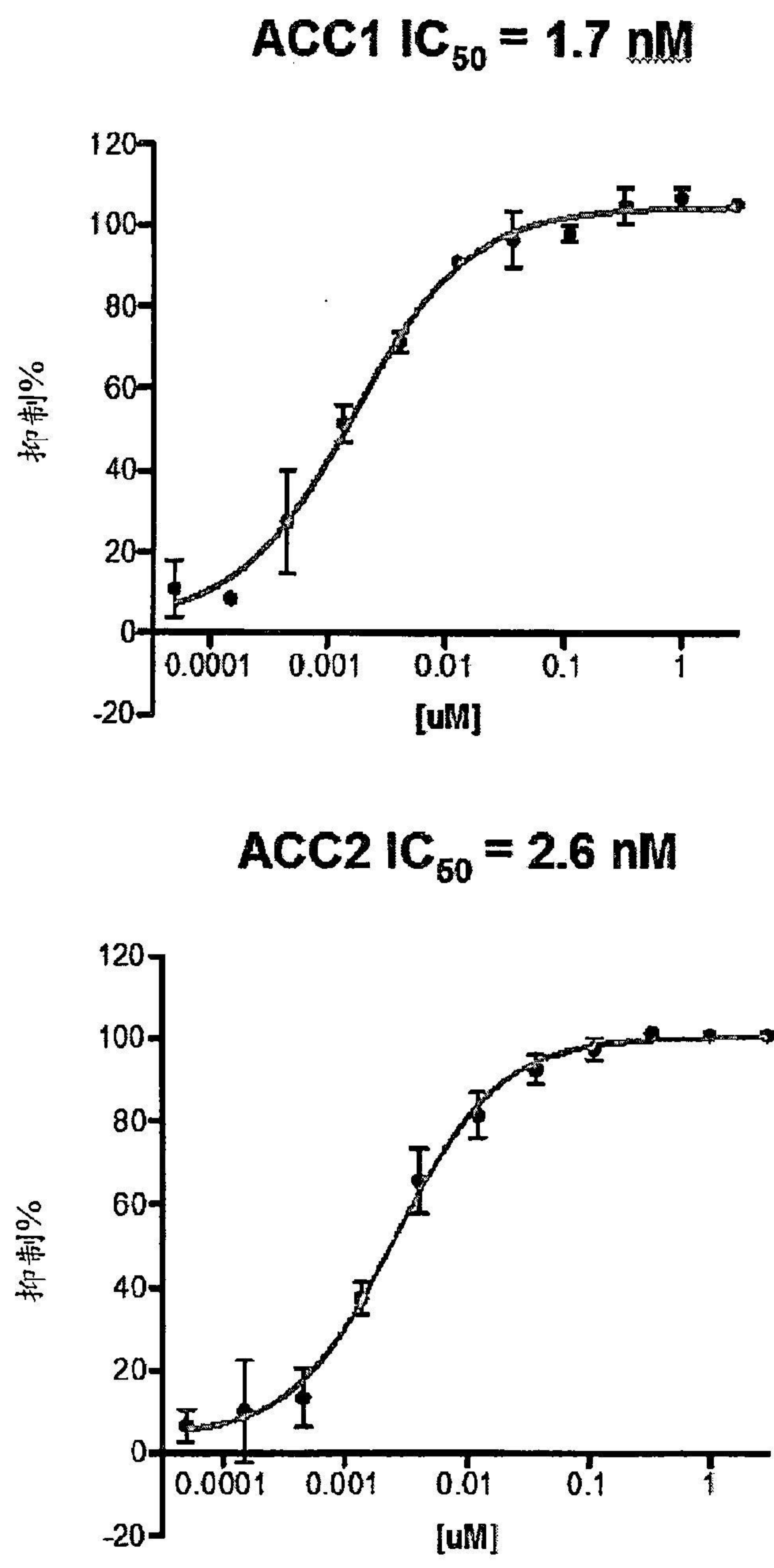
在活體外化合物I-181對ACC1及ACC2之酶抑制曲線。
