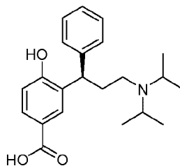
(VIIa)
