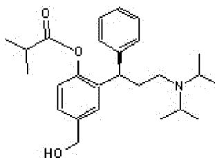
Fesoterodine
