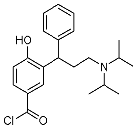
(IIa)
