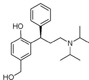
(Va)
