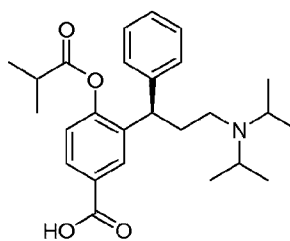
(VIIIa)
