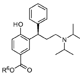
(IVa)
