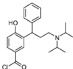
(IIa)
