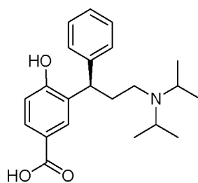
(VIIa)
