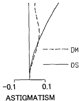
FIG. 15B (M-0.23m) Y'=3.3
