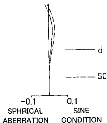
FIG. 14A (W-0.23m) FNO=2.59
