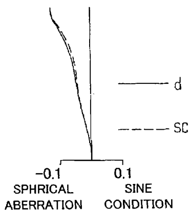
FIG. 15A (M-0.23m) FNO=3.29
