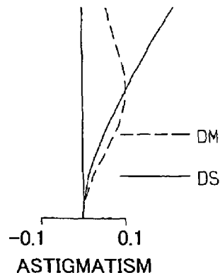
FIG. 16B (T-2.35m) Y'=3.3
