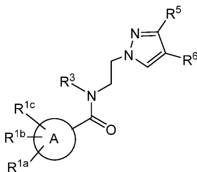
Ic
