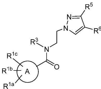
Ic
