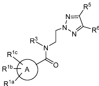
Ia
