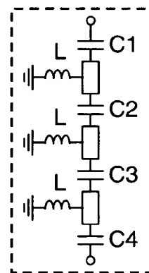
CRLH-TL FIG. 4B
