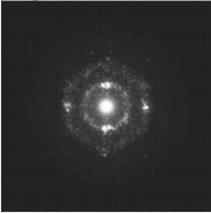
CAAC-OS
