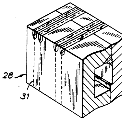
FIG. 8G
