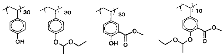
(RB-4) Mw 2500 Mw/Mn 1.4
