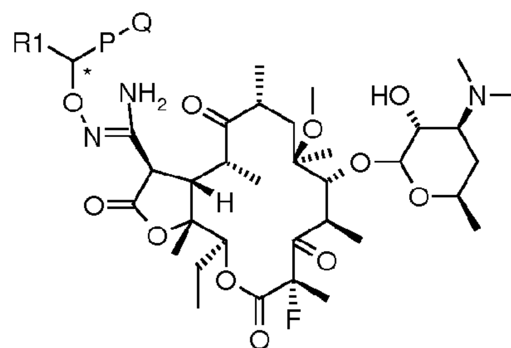
19-d' = R1 = CH 3
