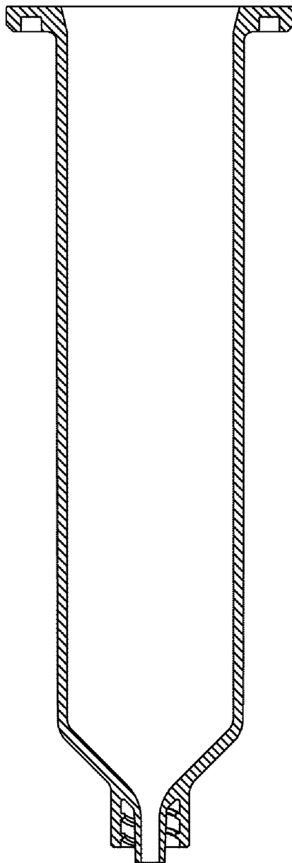
【A-A線剖面圖】
