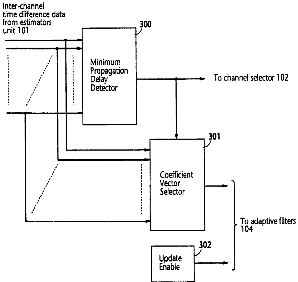
Controller 103
