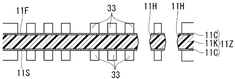
FIG. 4D
