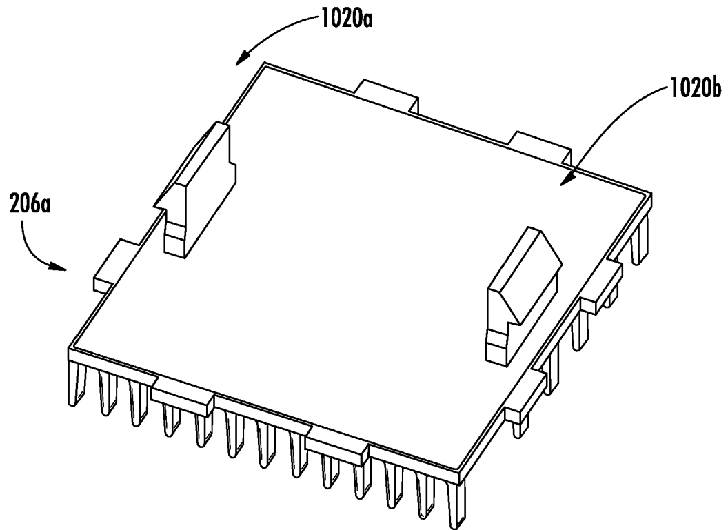
FIG. 10E
