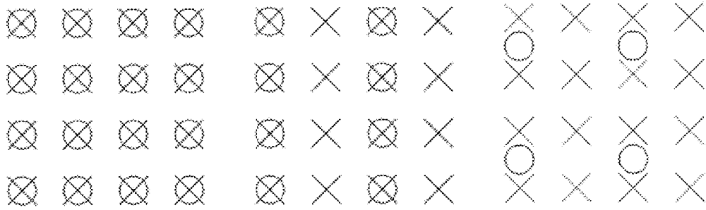
FIG. 1A - 4:4:4 format
