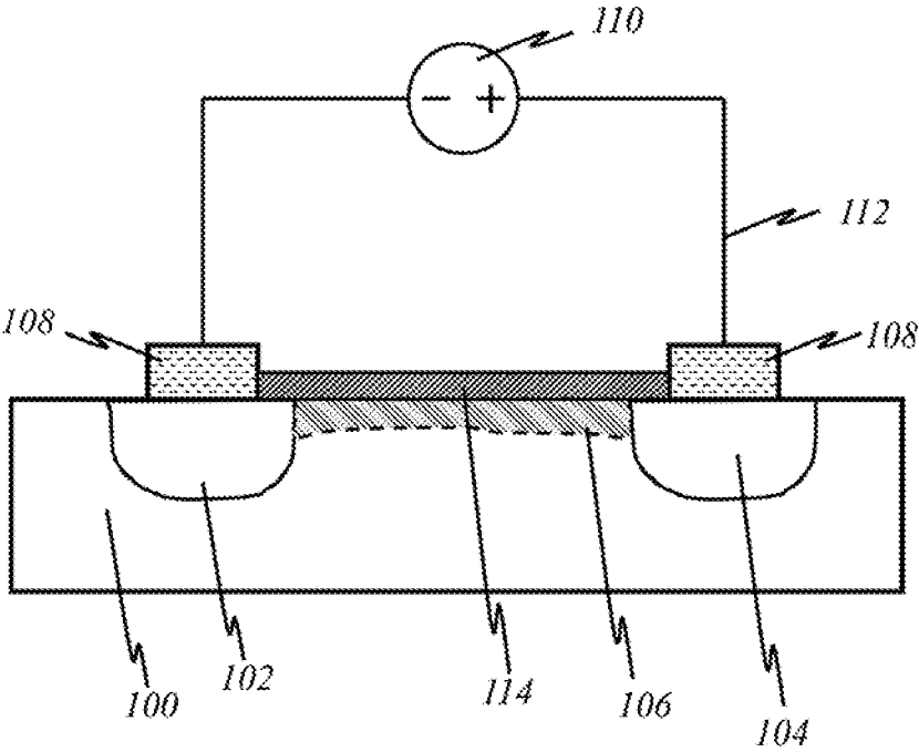
FIG. 1A Circuit
