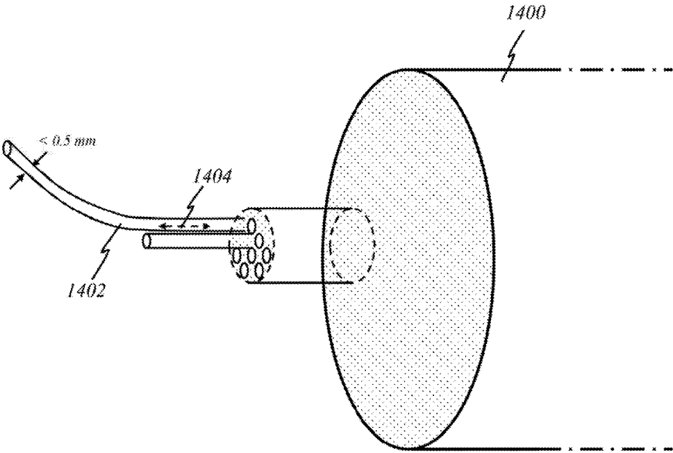
FIG. 13 Optical-fiber cable
