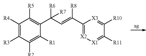
XXVIIIb
