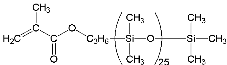
Silicone macromere (2)
