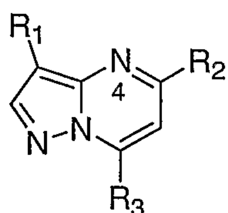
Pyrazolo[1,5-a]pyrimidines
