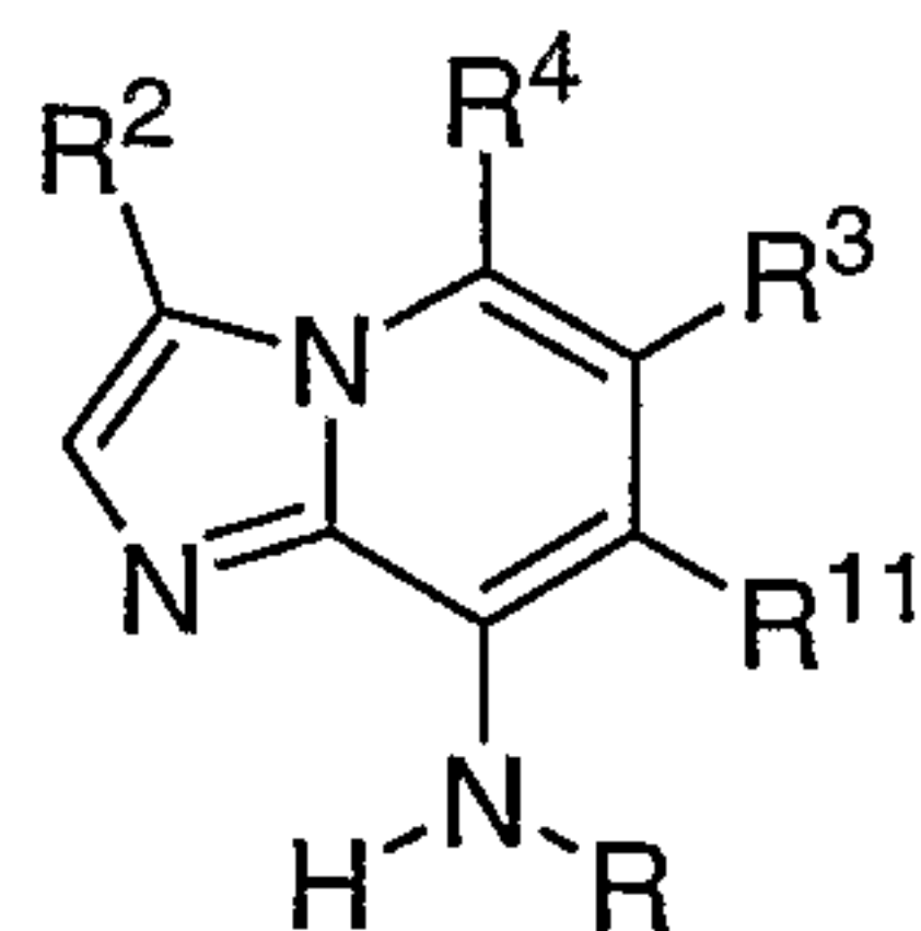
Imidazopyridine
