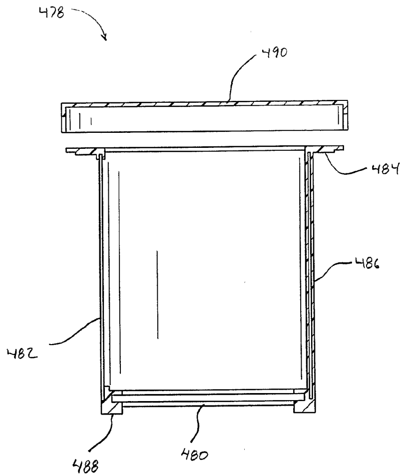
FIG. 49
