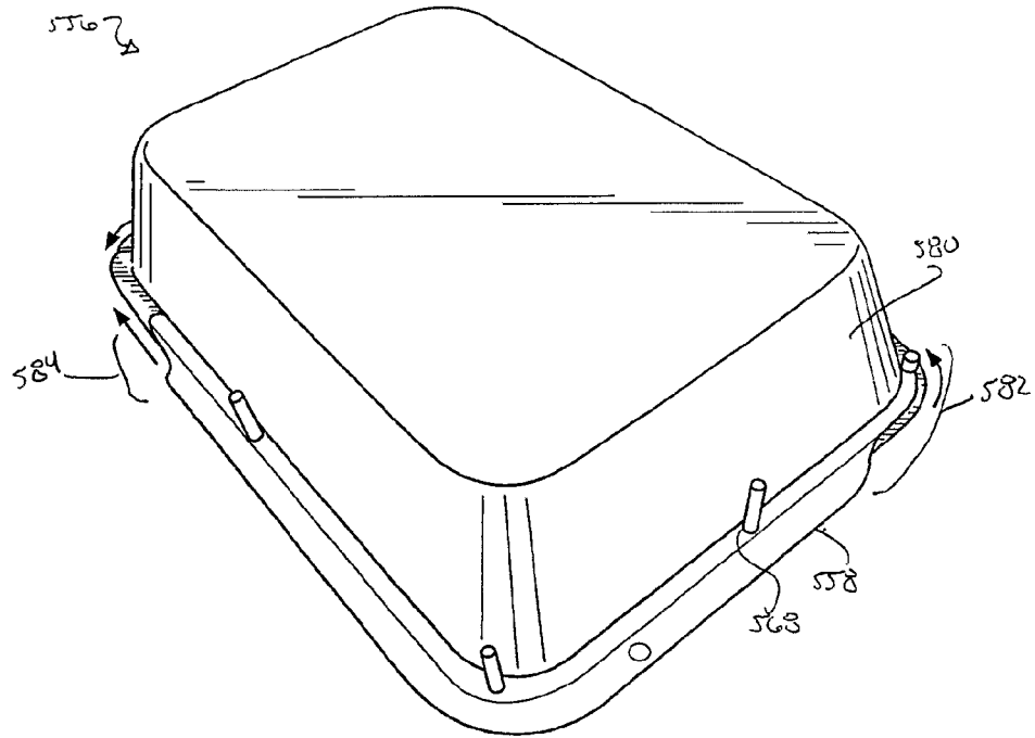
FIG. 67
