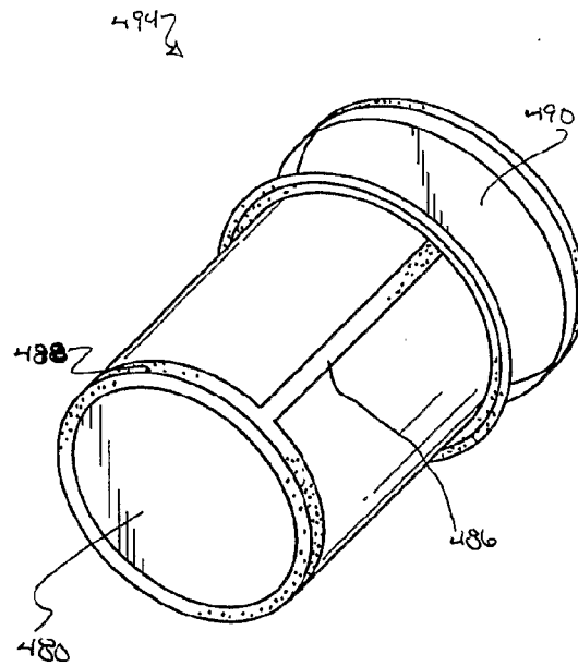
FIG. 50A
