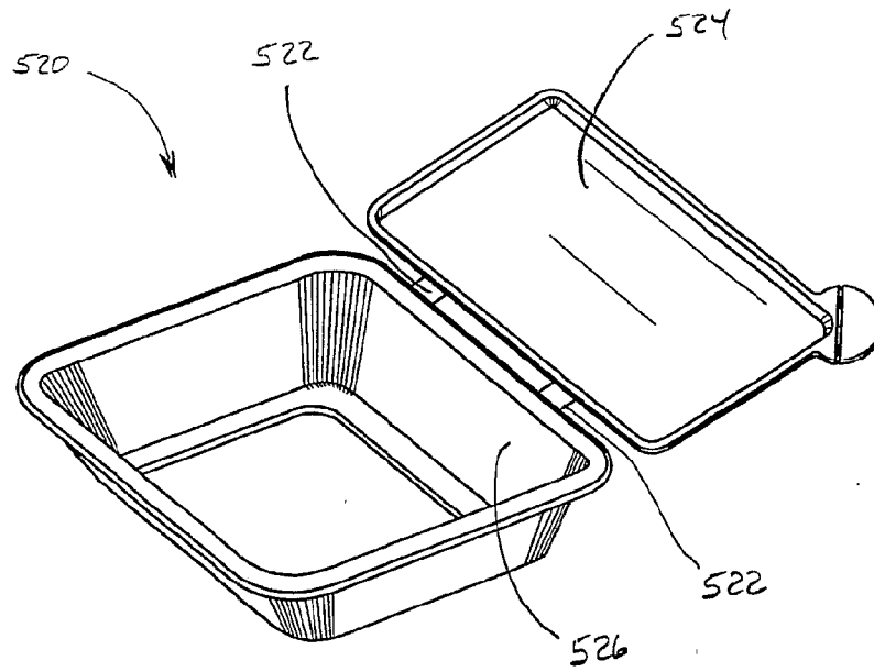
FIG.57
