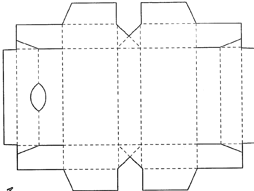
FIG. 44A
