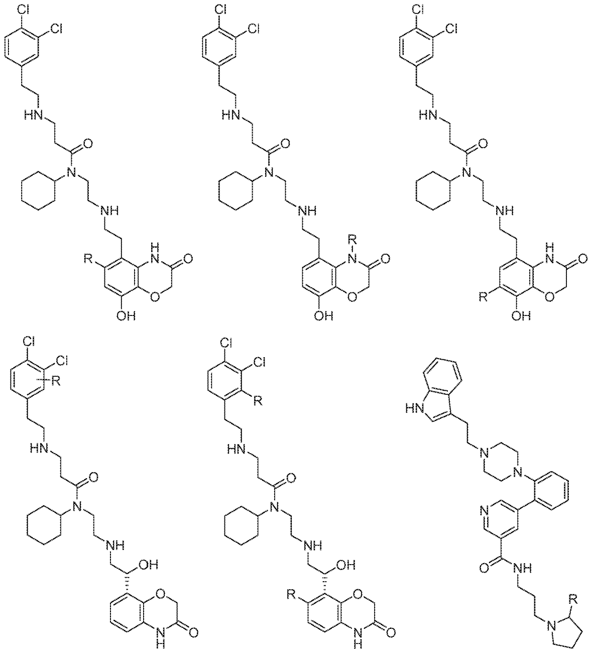
FIG. 4M
