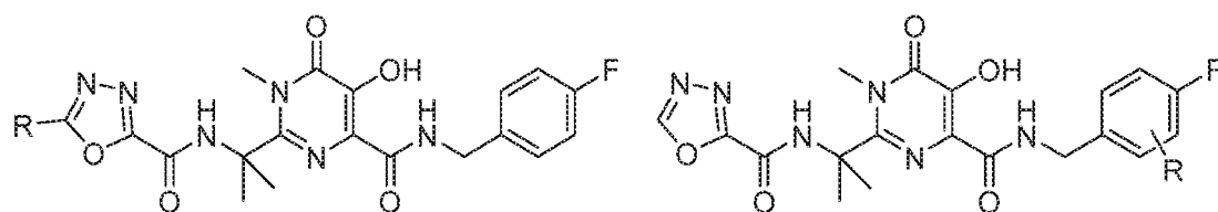
FIG. 1ZZ
