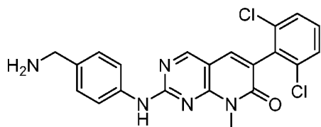
PD173955
