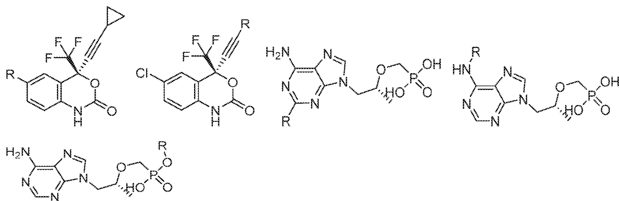
FIG. 3E
