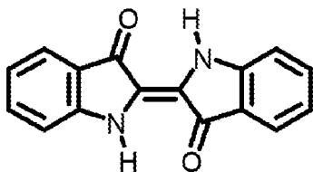
1H,1'H-[2,2']Biindolylidene-3,3'-dione
