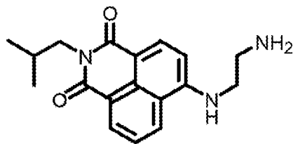
6-(2-aminoethylamino)-2-isobutyl-1H-benzo[de]isoquinoline-1,3(2H)-dione
