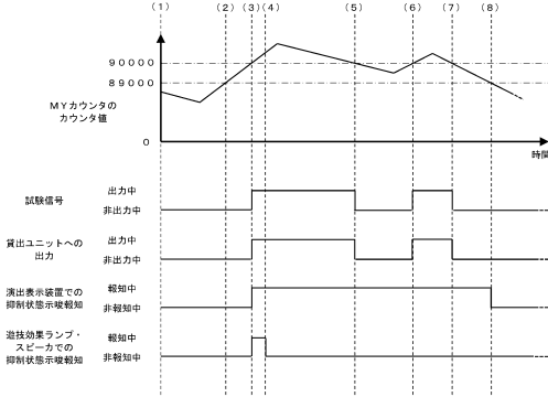
(図 4 9 2) <抑制状態示報報知に関する図>
