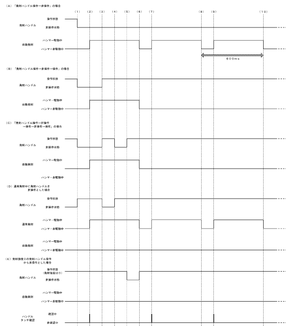
(図467) &lt;送付時の自動発射に関する作用図&gt;
