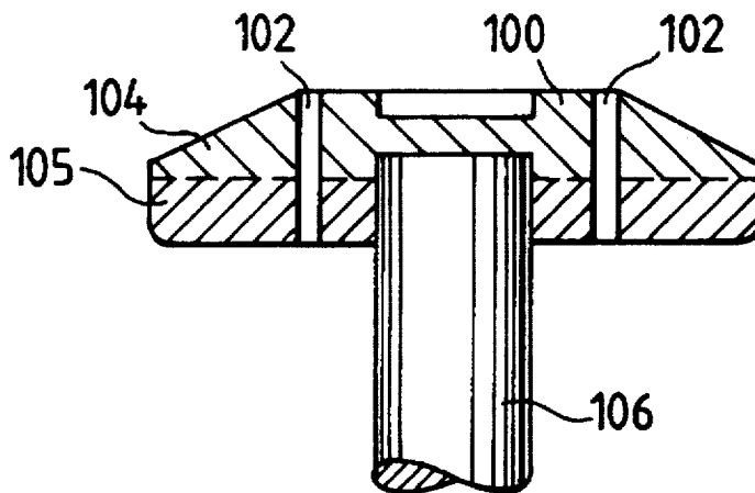
FIG. 14(b)
