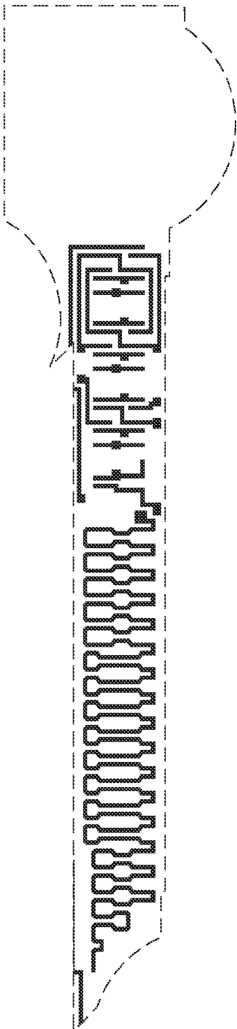
Poly mask
