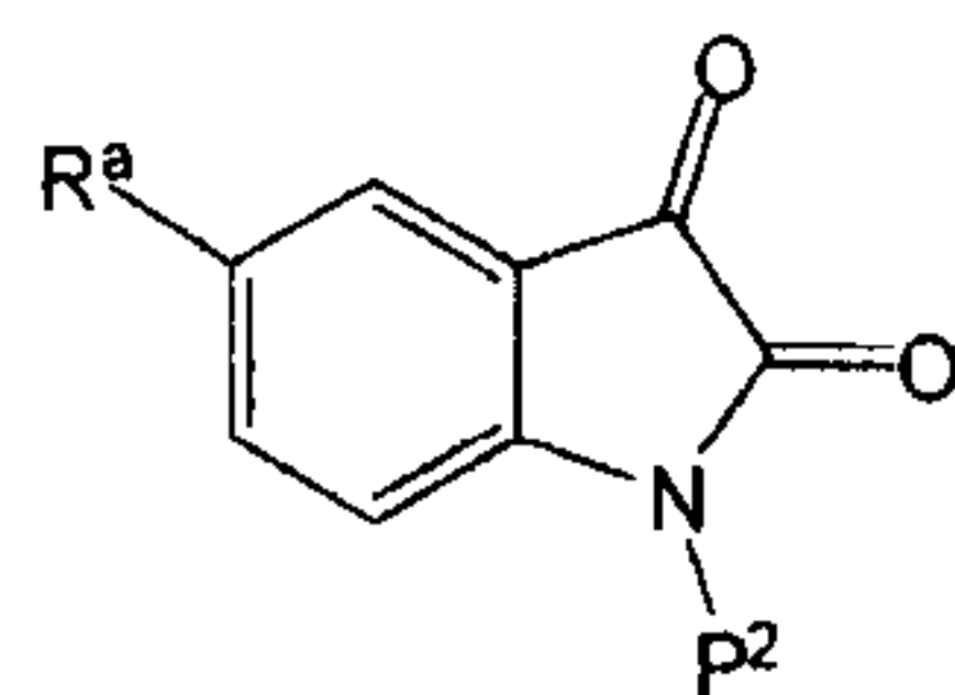
(VIIIa) ;
