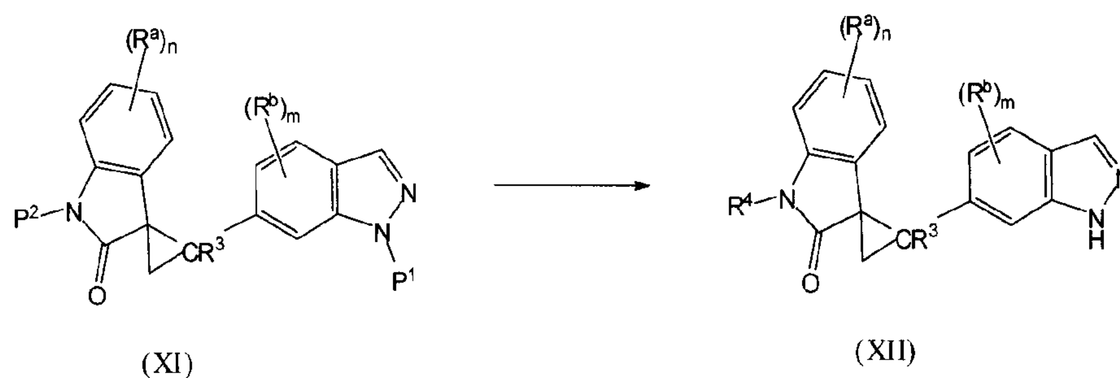
reaction 9a
