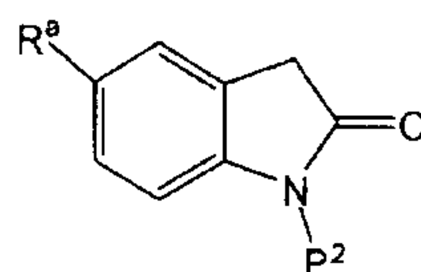
(Xa)
