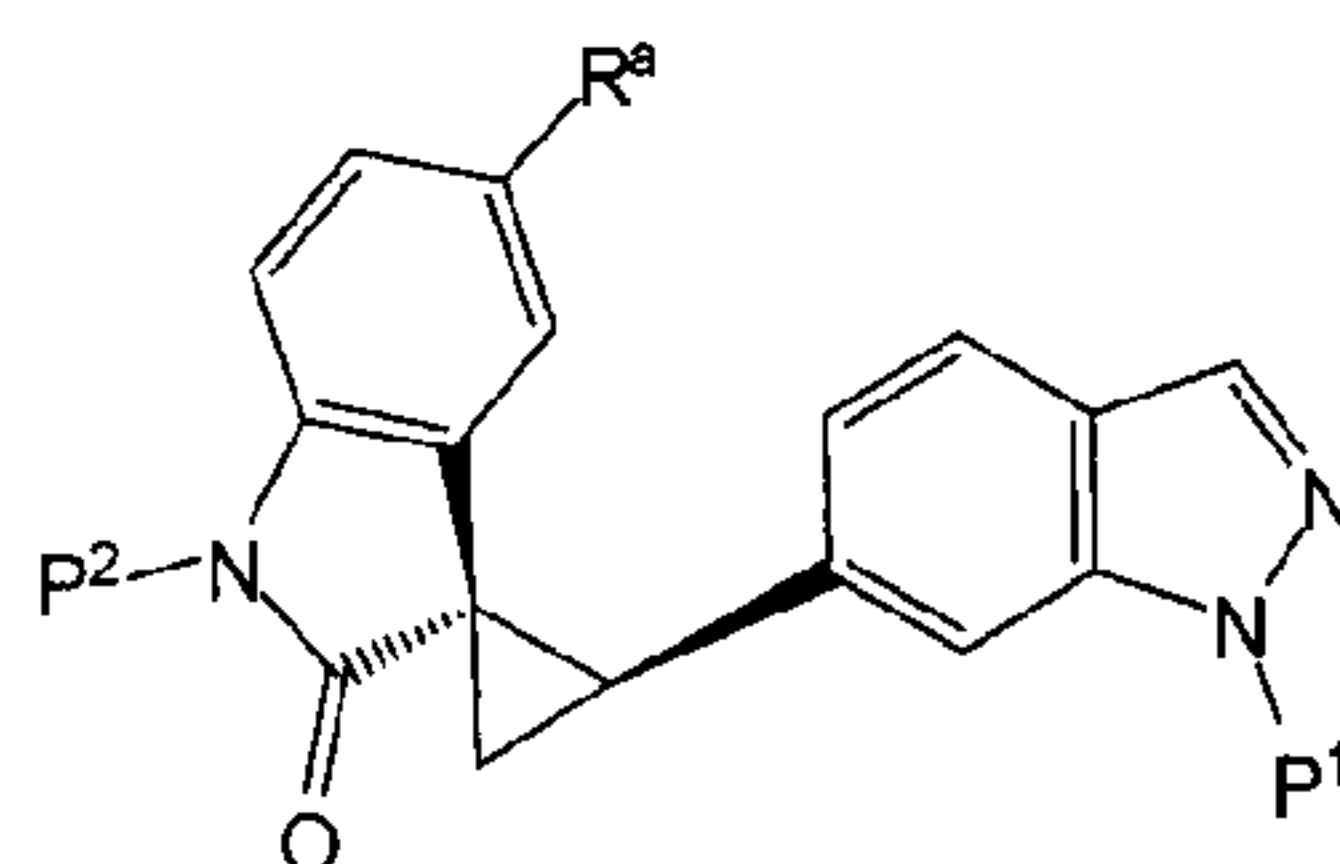
(XIc)
