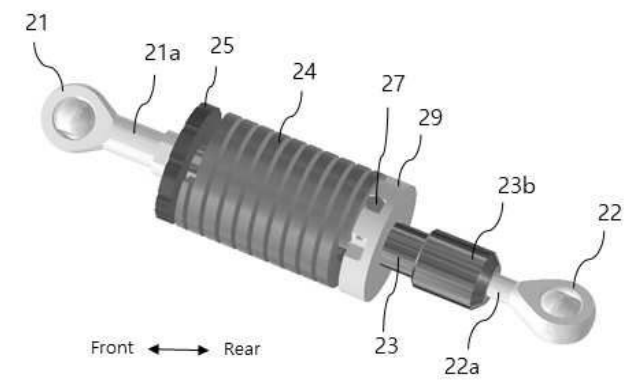
도면4
