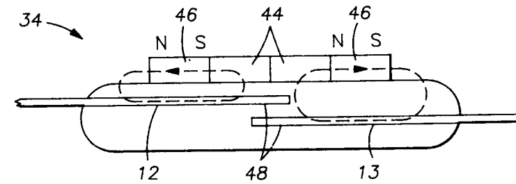
FIG. 6C
