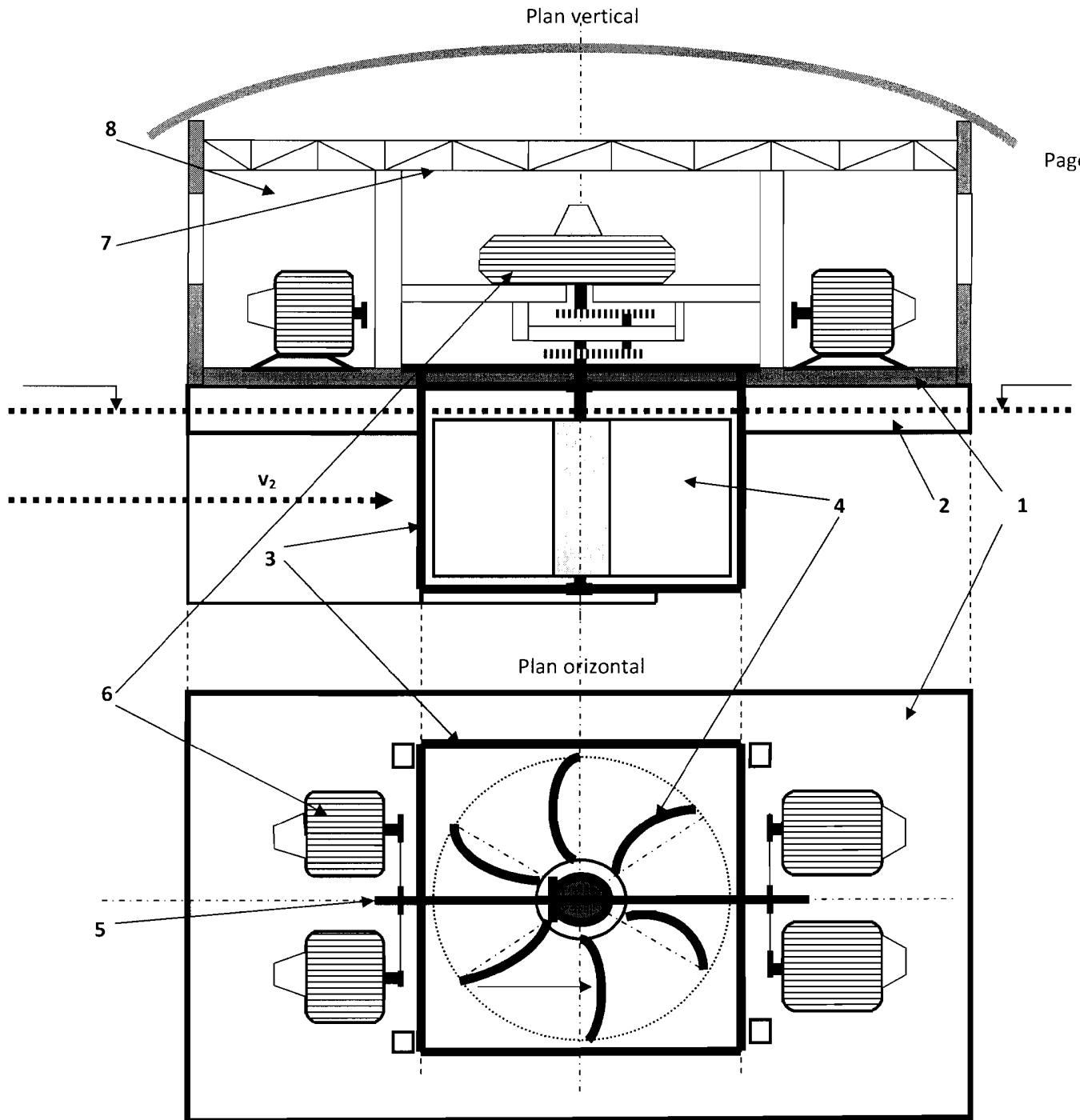
Fig.nr.9/9 : Hidro Tornado Electrica – in functiune.
