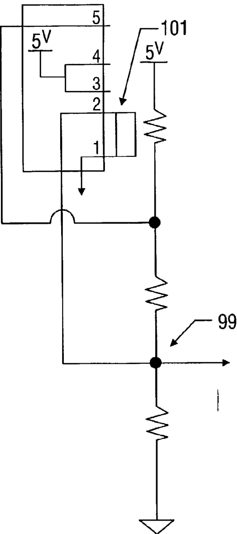
FIG. 9B
