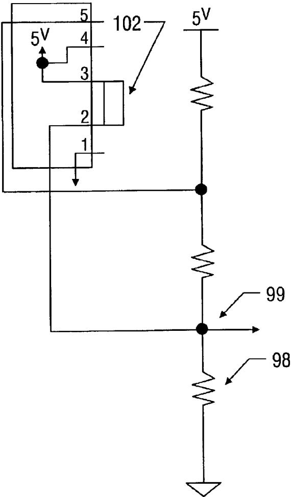
FIG. 9C
