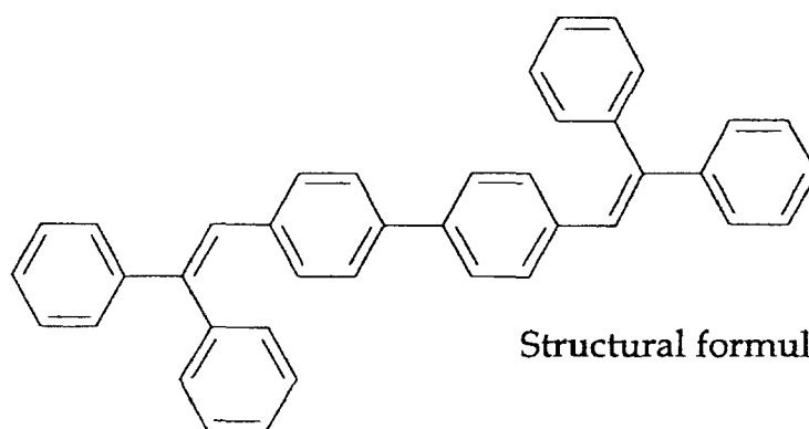
DPVBi
