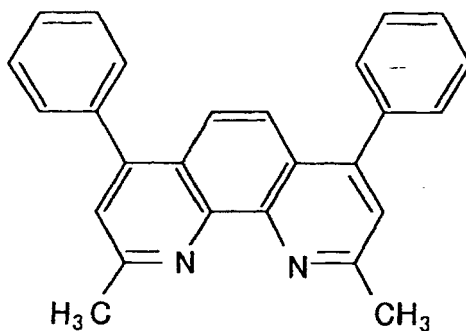
BCP
