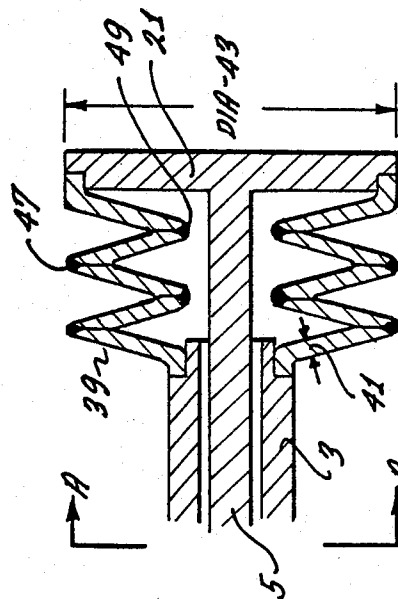
Fig. 3 (METAL DIAPHRAGM)
