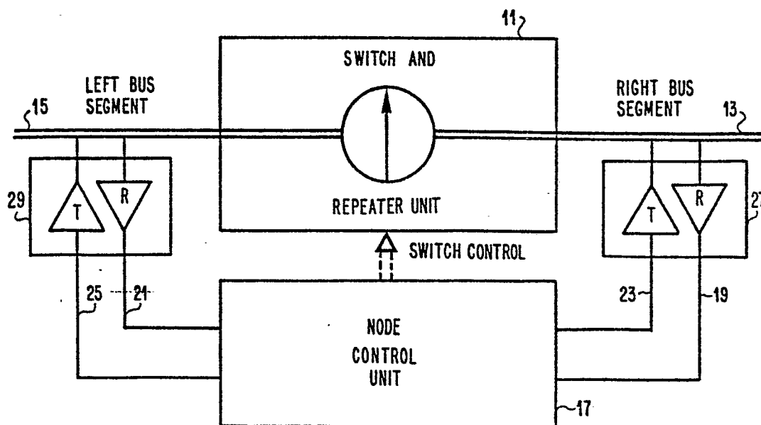
FIG. 2 NODE
