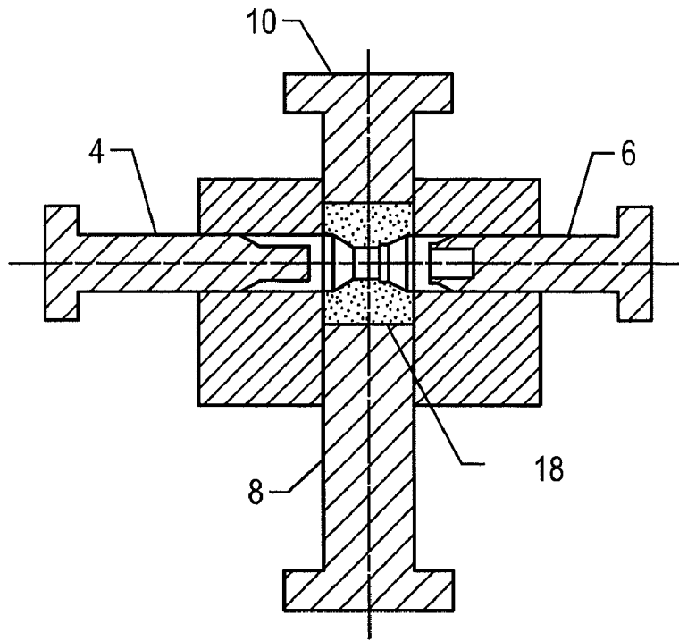
FIG. 3G
