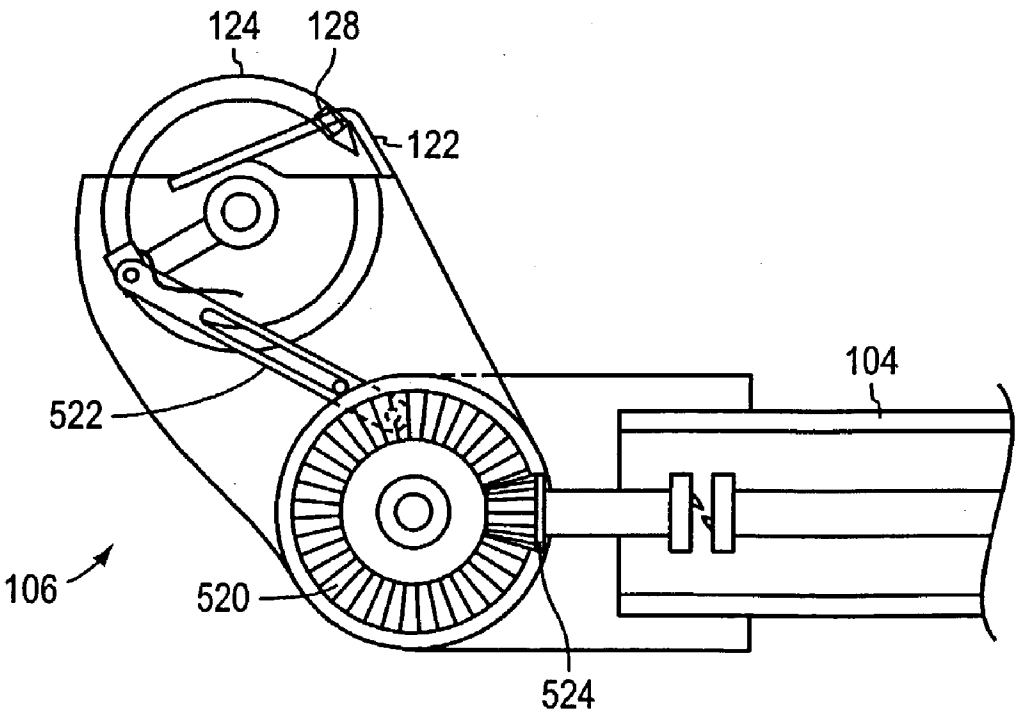
FIG. 9C
