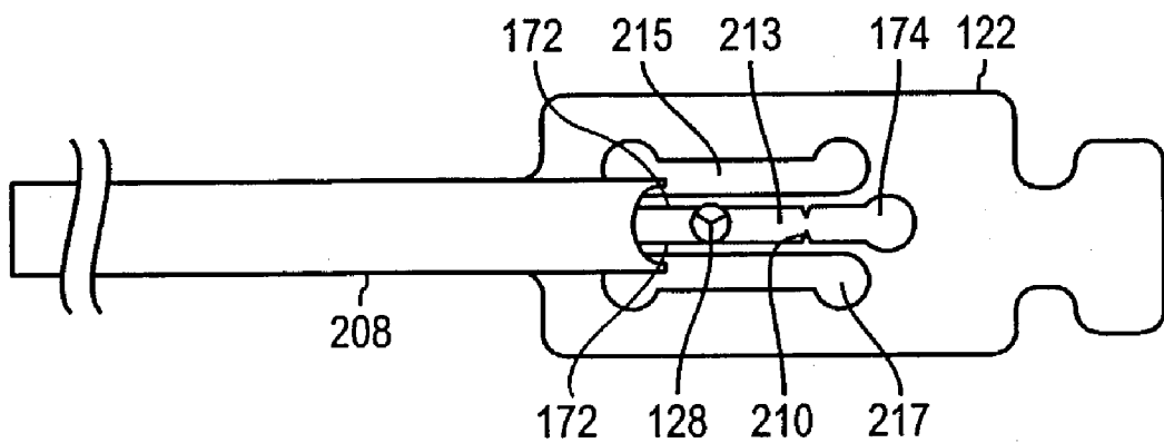
FIG. 5D
